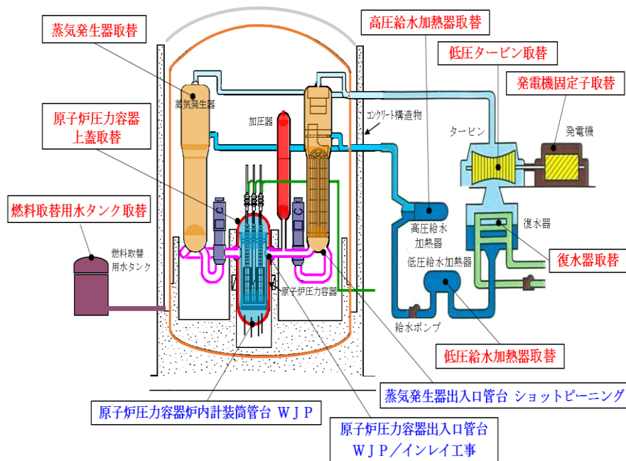
(PWRプラントの例)
