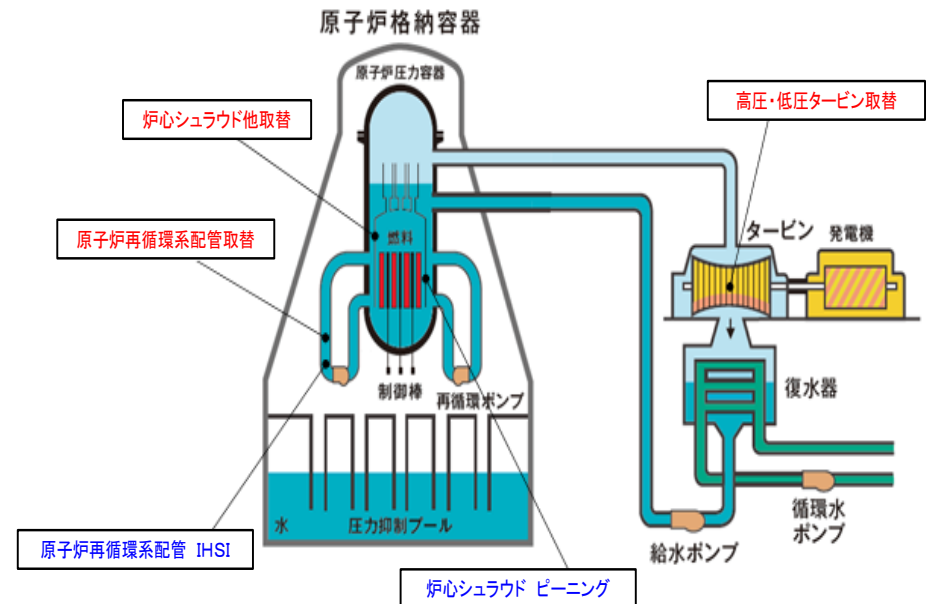
(BWRプラントの例)
